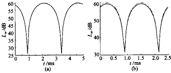
图 4 根据第 1 阶辐射模态计算的声功率 Fig. 4 Sound power in first radiation mode (a) f=200\text{ Hz} (b) f=400\text{ Hz}
